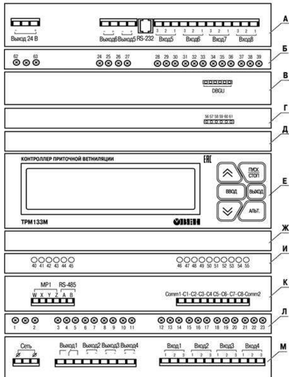
Рисунок 3.1 – Прибор ТРМ133М-02: внешние связи, элементы индикации и управления
